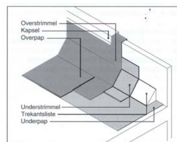
Figur 8.2.1: Inddækning af stern med to-lags inddækning og kapsel.
